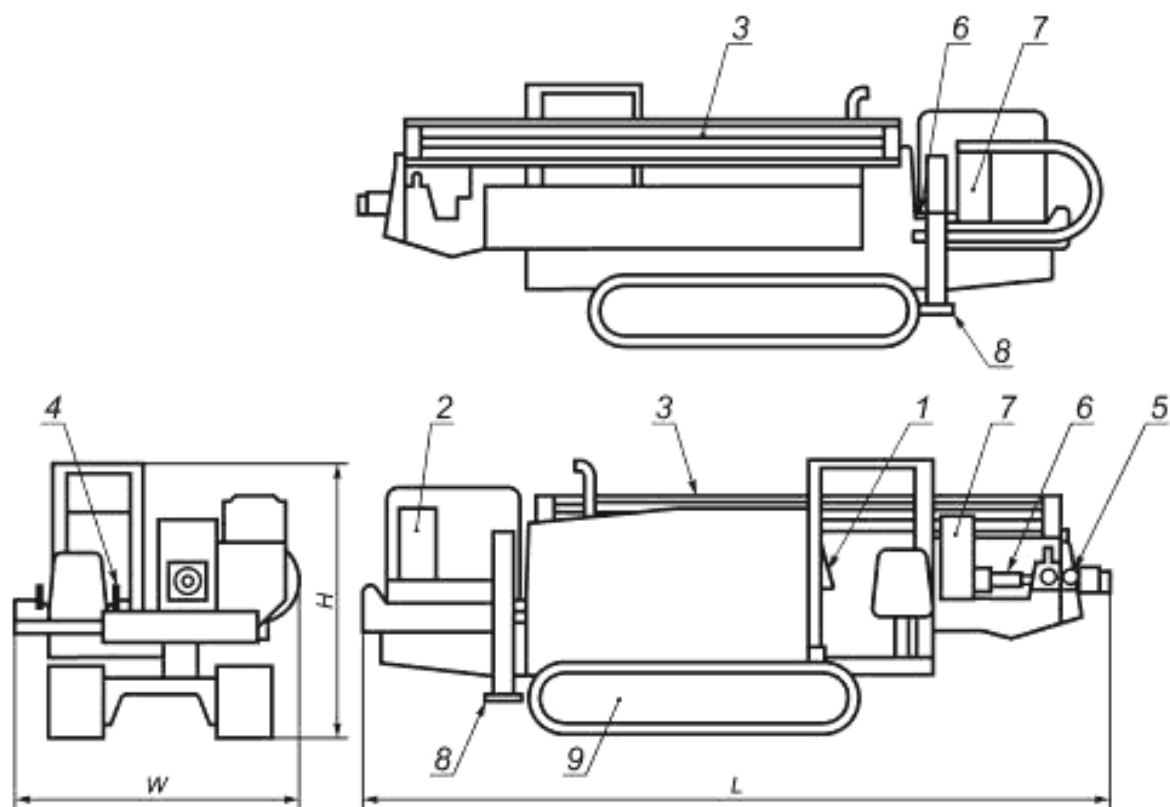
H — общая высота машины; L — общая длина машины; W — общая ширина машины; 1 — управление установкой машины; 2 — бак для воды; 3 — ящик для буровых труб; 4 — управление процессом бурения — место оператора; 5 — зажим; 6 — шпindel; 7 — каретка; 8 — задний аутригер; 9 — шасси
