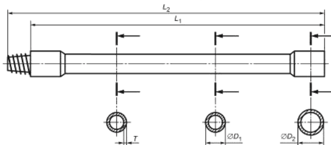
Рисунок 5 — Бурильная труба
