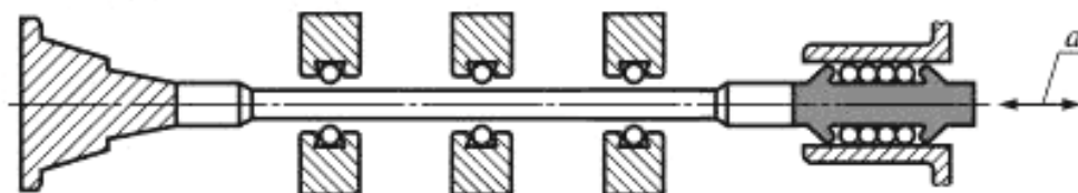
Рисунок 8 — Бурильная труба. Испытание по определению толкающего/тянущего усилия
