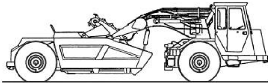
Рисунок А.2 — Колесный скрепер с элеватором
