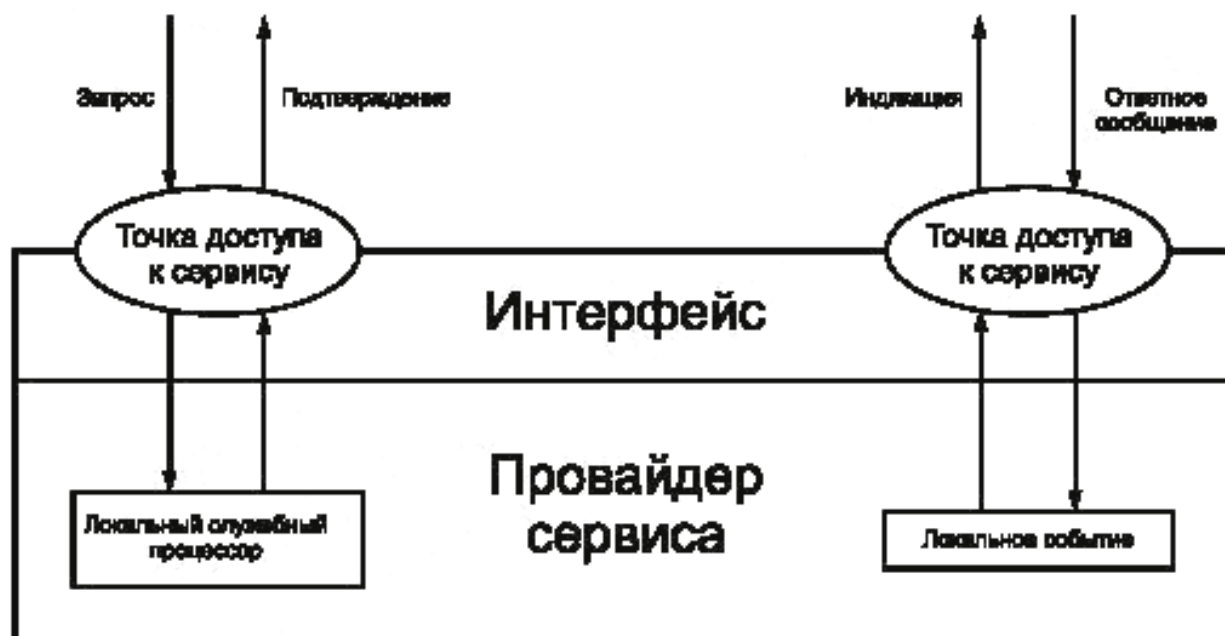
Рисунок 1 — Обработка локальных событий с помощью VDS-сервиса
