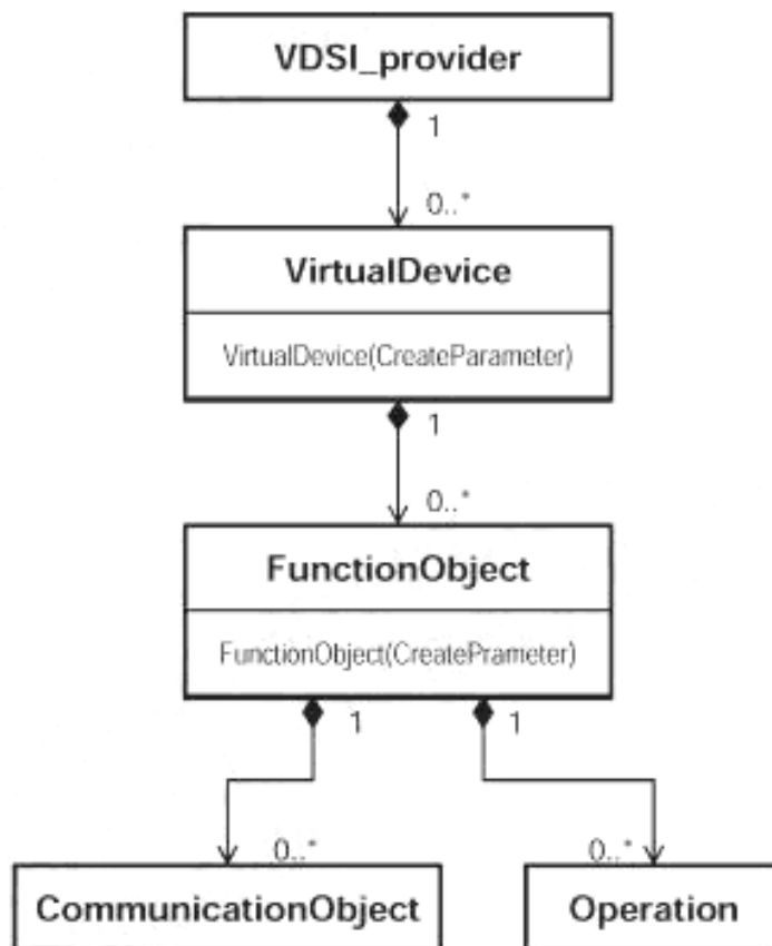
Рисунок 3 — Диаграмма UML-класса VDSI-модели
