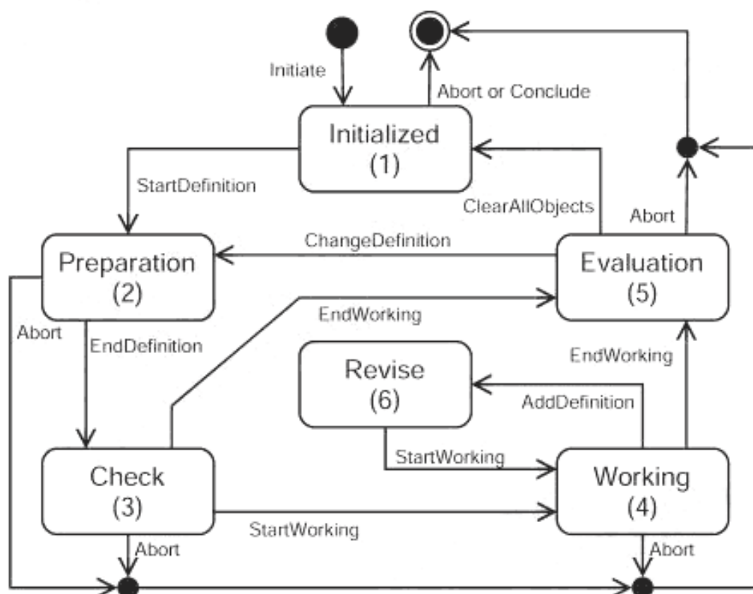
Рисунок 6 — Рабочие состояния виртуальных устройств
