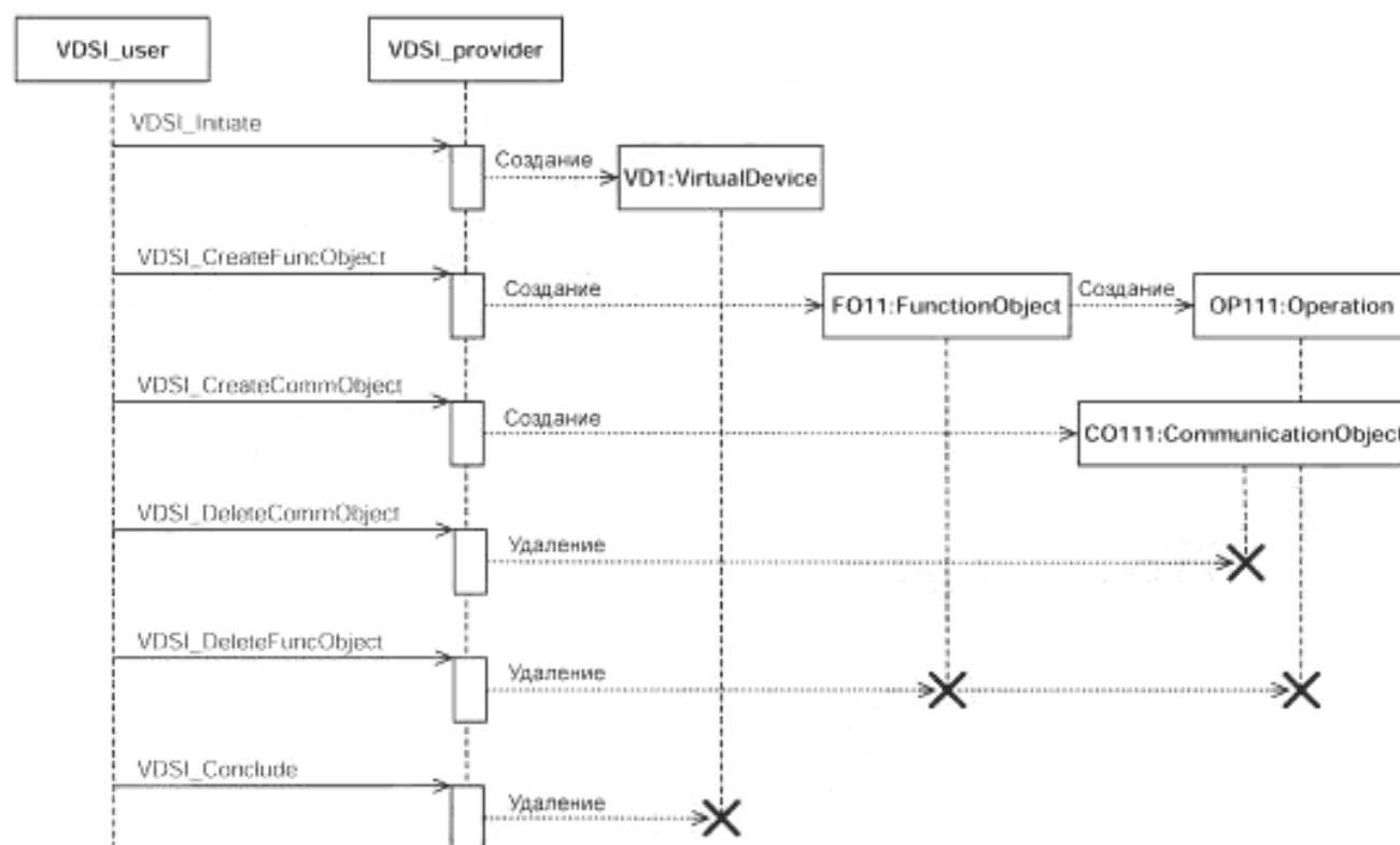
Рисунок 4 — UML-схема последовательности операций для продолжительности жизни VDSI-объектов
