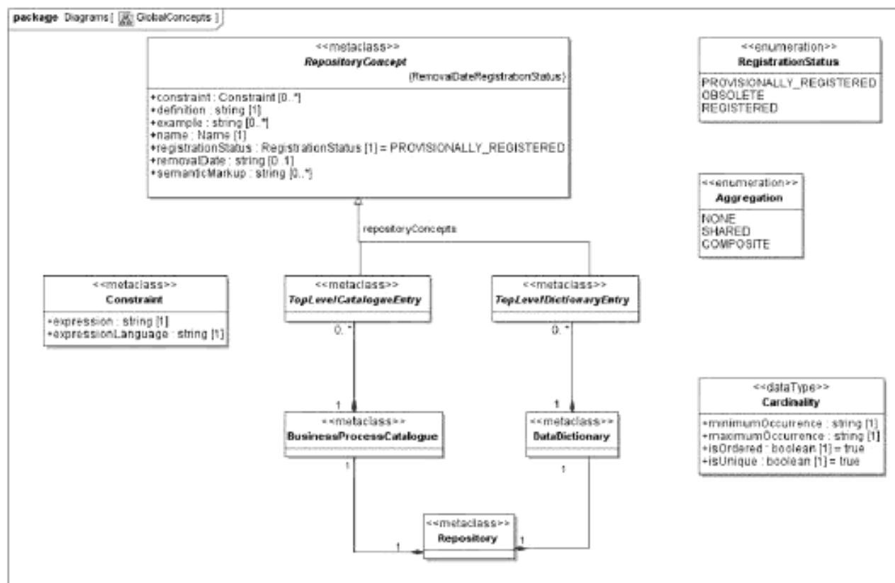
Рисунок 13 — Глобальные концепты
