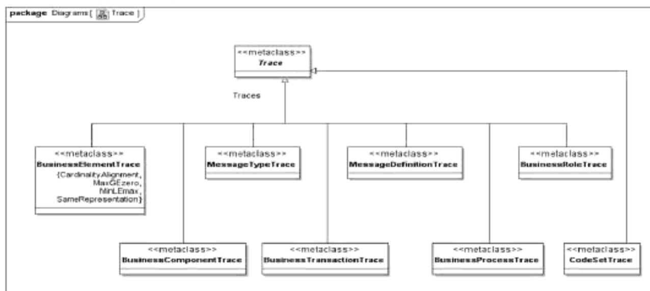
Рисунок 9 — Следы
