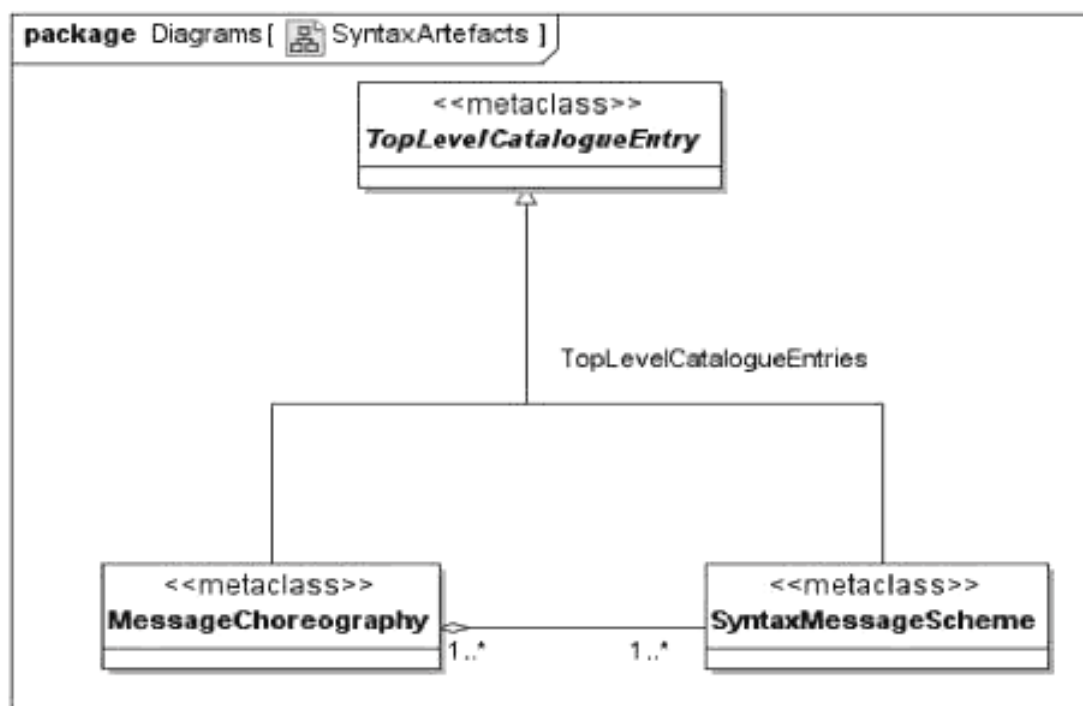
Рисунок 8 — Синтаксис артефактов
