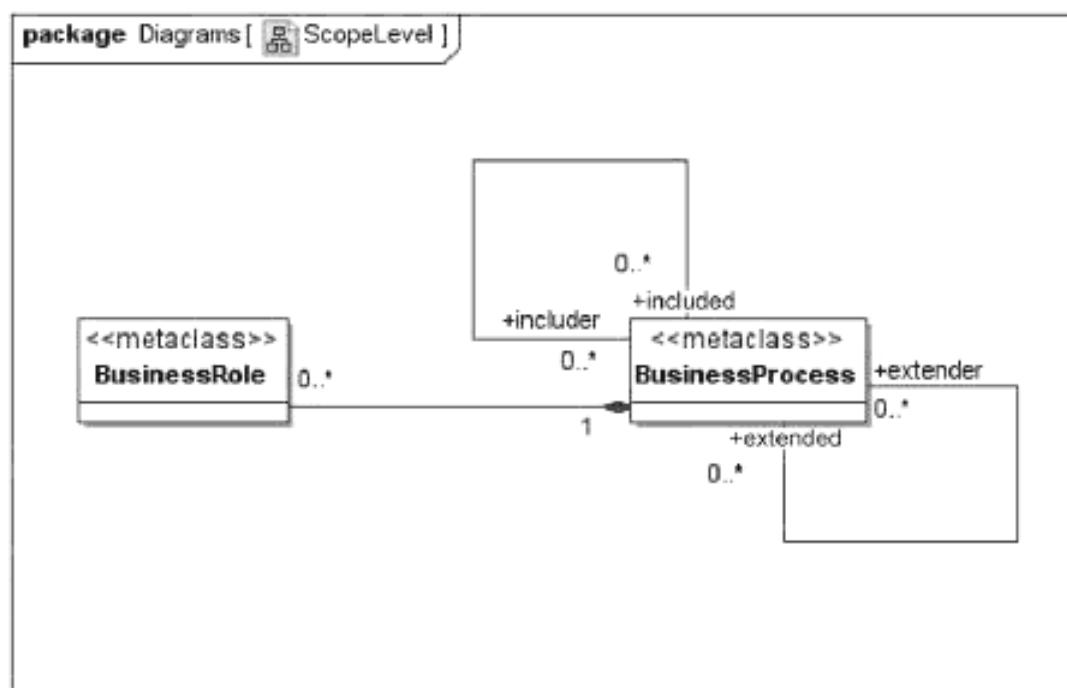
Рисунок 4 — Обзорный уровень
