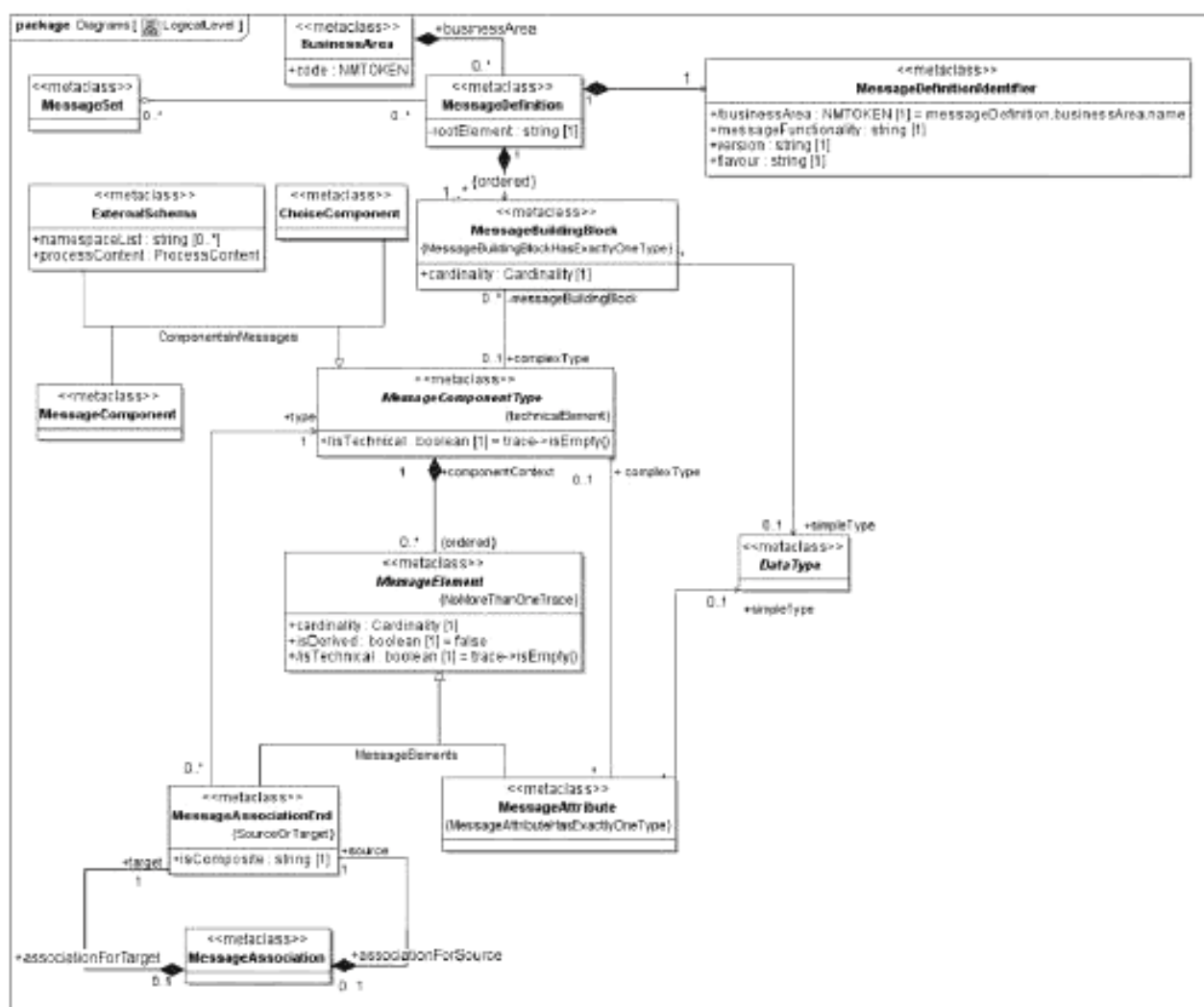
Рисунок 7 — Логический уровень
