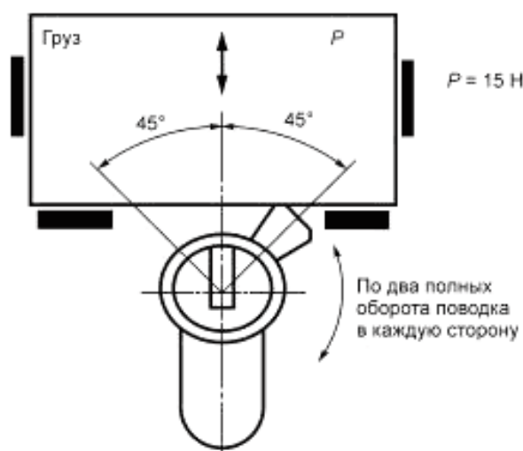
Рисунок 1 — Схема испытания цилиндрического механизма наработку
