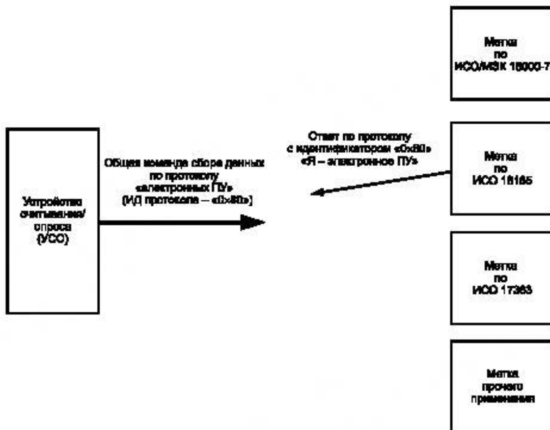
Рисунок А.1 — Запрос и ответ по конкретному идентификатору протокола
