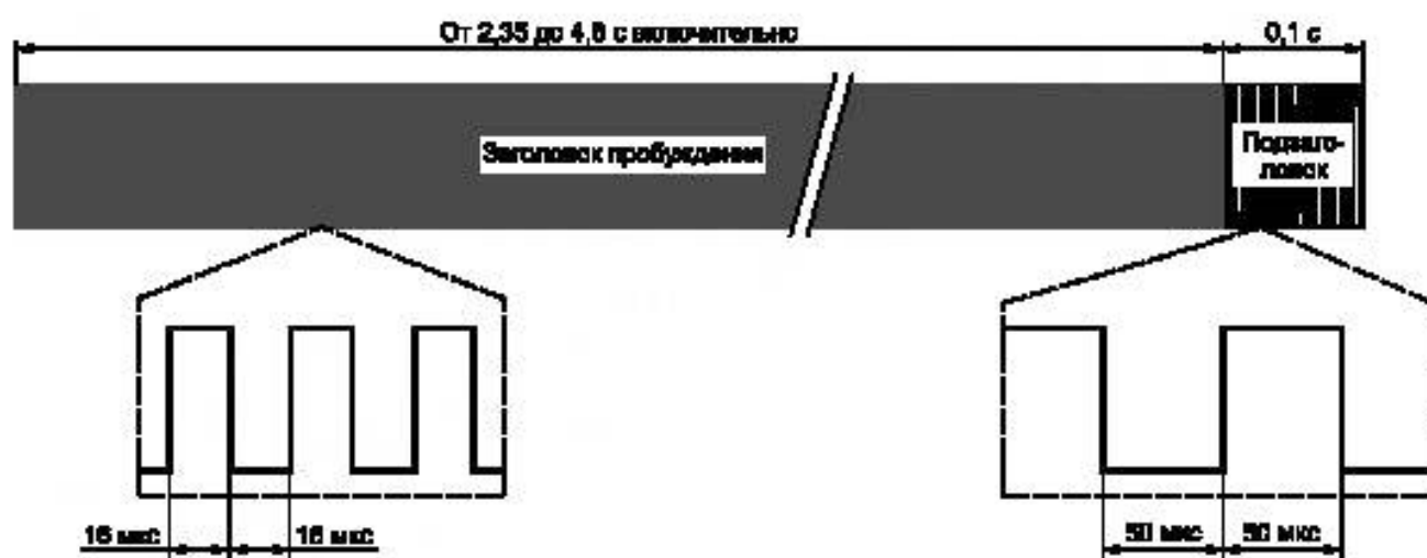
Рисунок 1 — Сигнал пробуждения «Wake Up»
