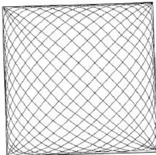
Рисунок 1 – Фигура Лиссажу
