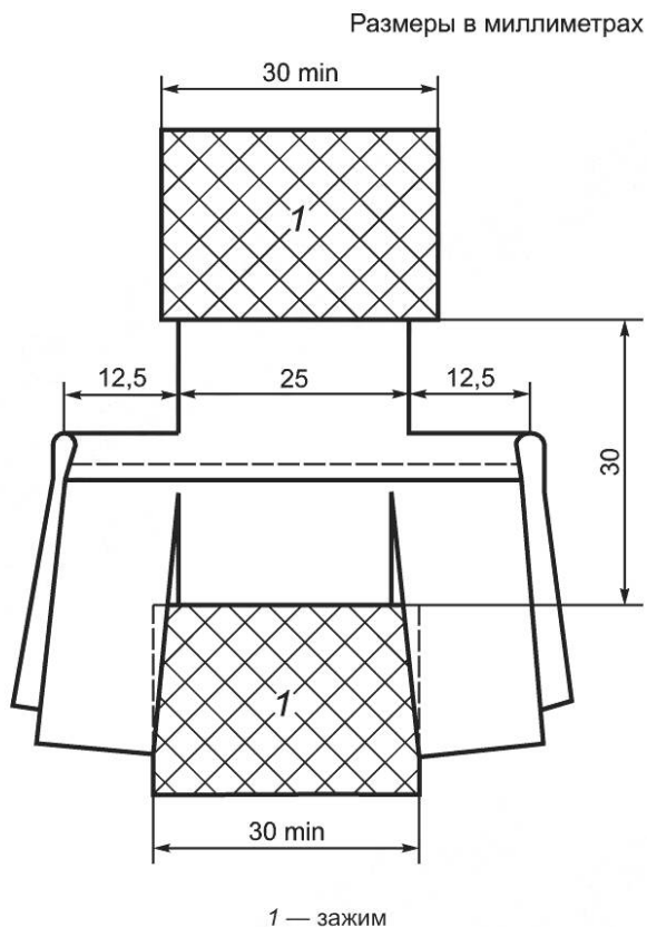
Рисунок 4 — Зажатая испытываемая проба
