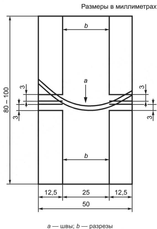
Рисунок 3 1) — Испытуемая проба, вырезанная из обуви
