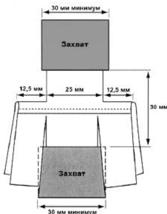
Рисунок 4 — Испытуемый образец в захватах
