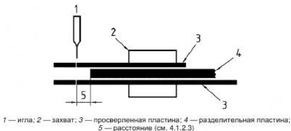
Рисунок 1 — Схематическое изображение устройства с иглой
