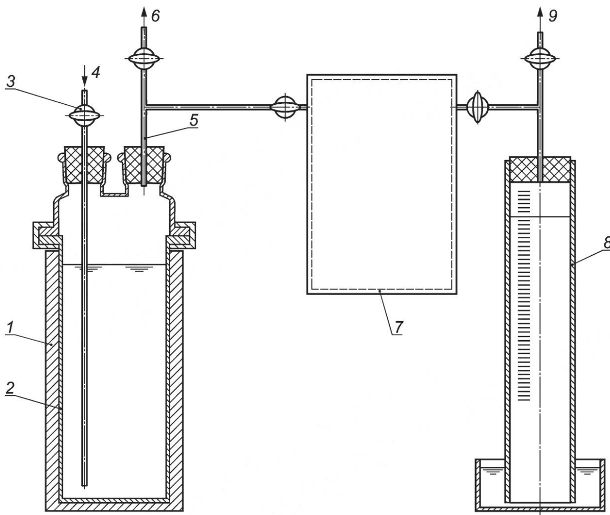
1 — термостатируемая баня; 2 — сосуд для ферментативного разложения; 3 — клапан; 4 — подача газа N_2 ; 5 — выход газа; 6 — выпуск газа N_2 ; 7 — мешок для сбора газа; 8 — газовая бюретка; 9 — выпускной клапан
