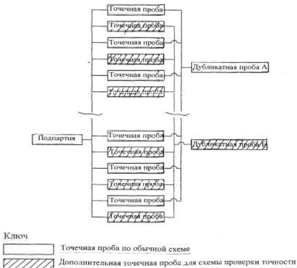
Рисунок 1. Пример плана дубликатного опробования
