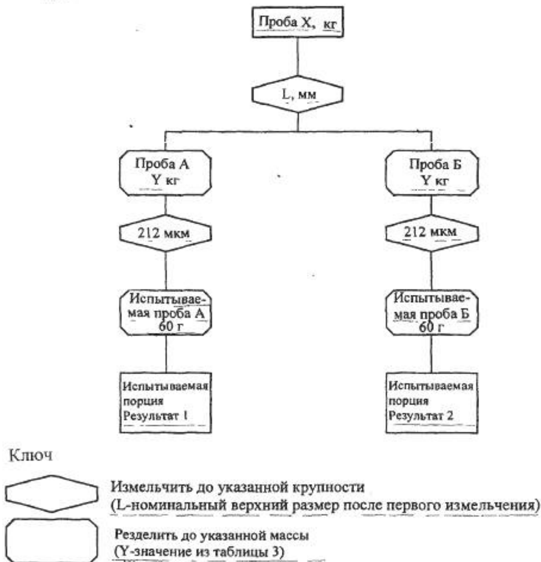
Рис. 3 Полное испытание подготовки проб
