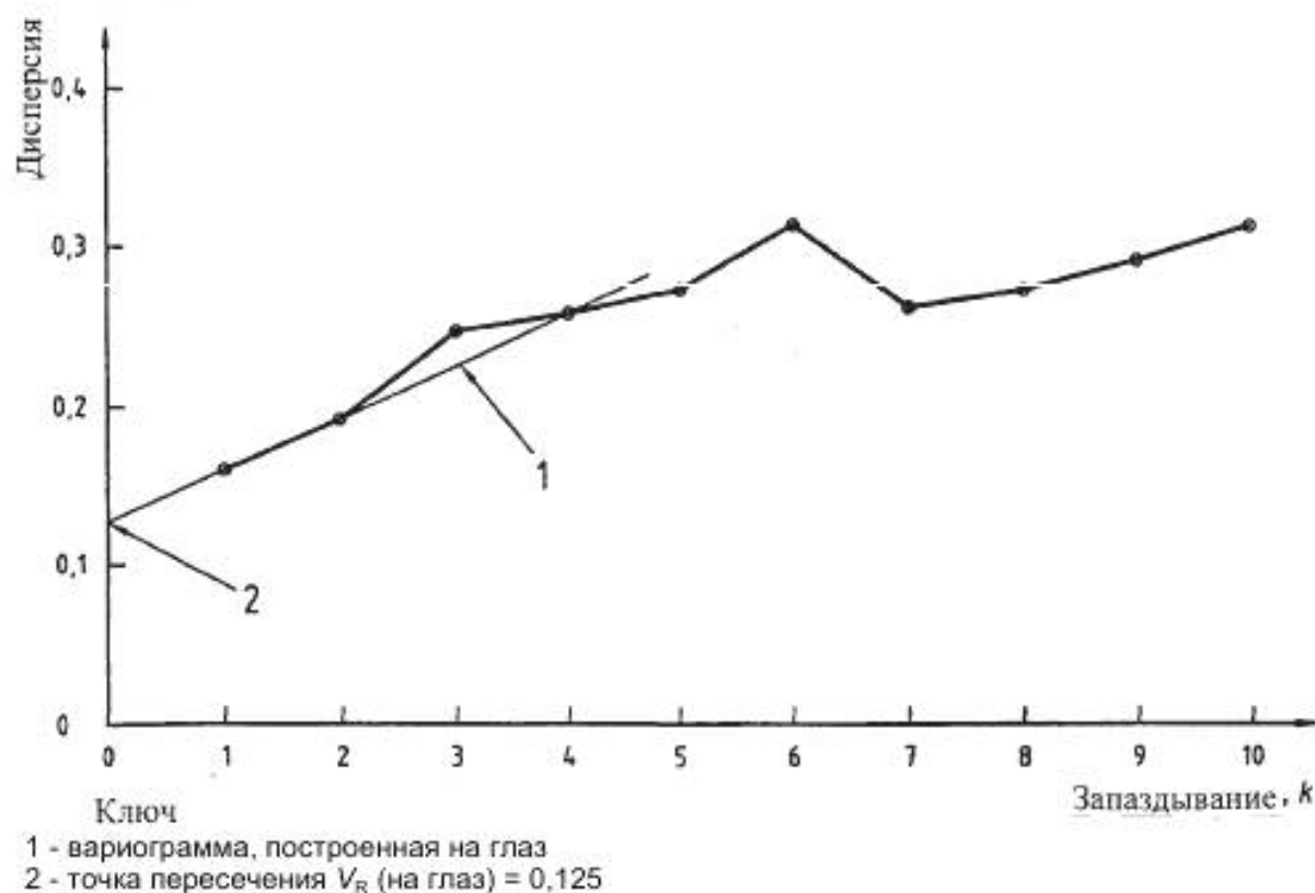
Рисунок 3 Вариограмма для данных из таблицы А.2
