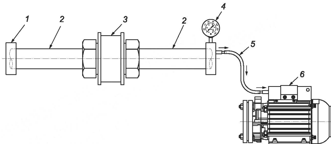
1 — концевая заглушка; 2 — участок трубы; 3 — испытуемый узел; 4 — вакуумметр; 5 — подключение к вакуумному насосу (запорный вентиль не изображен); 6 — вакуумный насос
