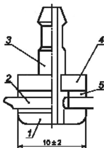
Рисунок 1 — Штуцер
