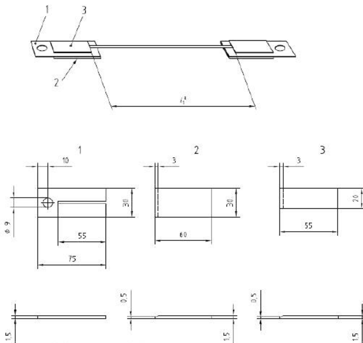
Рисунок С.4 — Петли из металлического листа
