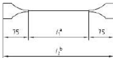
Рисунок С.1 — Термопластмассовые петли
