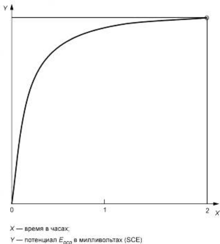
Рисунок 3 — Зависимость потенциала разомкнутой цепи от времени
