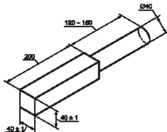
Рисунок 6 — Уплотняющий брус
