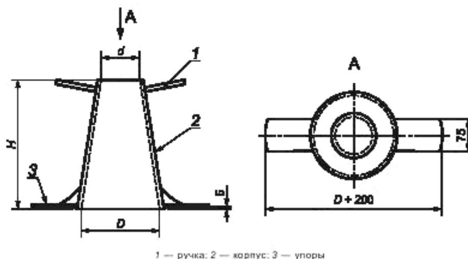
Рисунок 1 — Конус для определения подвижности
