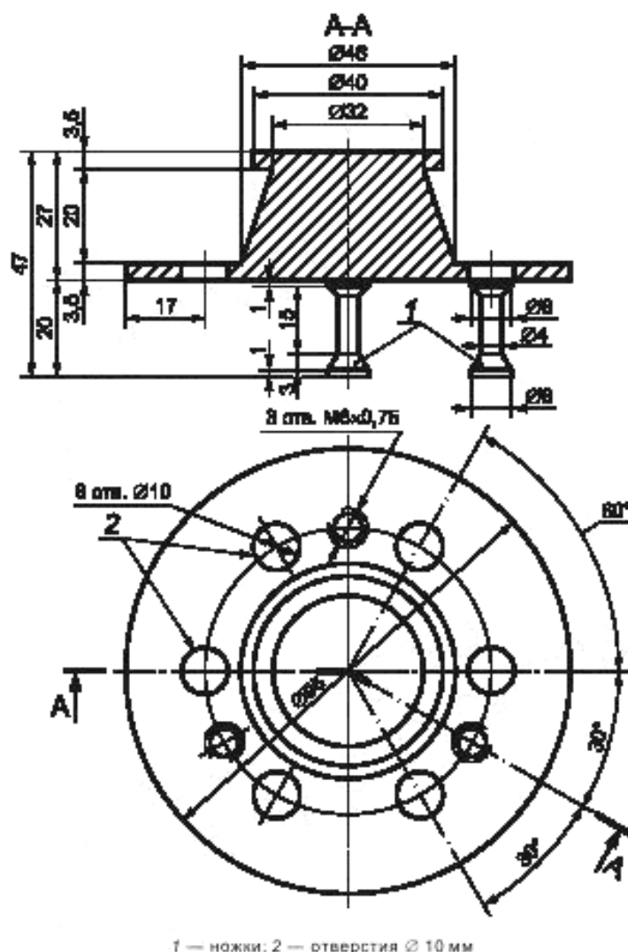
Рисунок 3 — Прибор Красного
