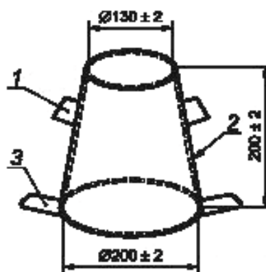
1 — ручка; 2 — корпус; 3 — упоры
