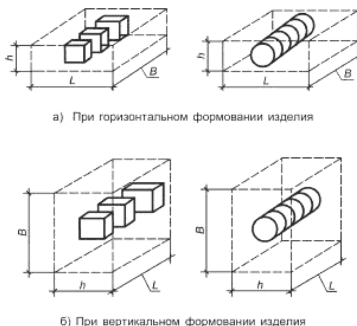
Рисунок 1 — Схемы выпиливания и выбуривания образцов ячеистого бетона
