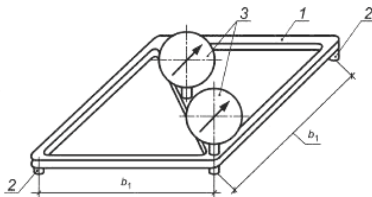
b_1 — база прибора; 1 — корпус (рамка); 2 — опора; 3 — индикатор
