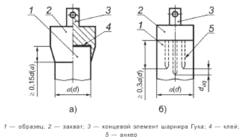
Рисунок К.2 — Схема приклеиваемых и анкерных захватов
